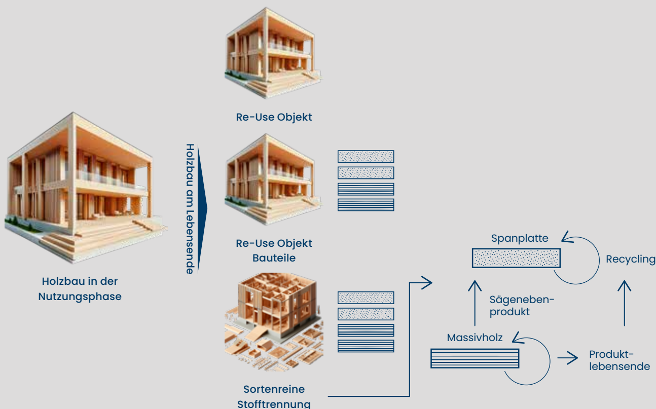
Abbildung 3: Mögliche Verwertungswege von Holzgebäuden und Bauprodukten am Lebensende (aus dem Englischen übersetzt von 13 )
