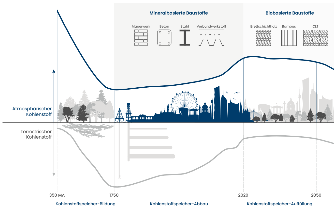
Abbildung 2: Darstellung von Prozessen für die Bildung, den Abbau und die Auffüllung von Kohlenstoffspeichern, angelehnt an Churkina et al. 12
