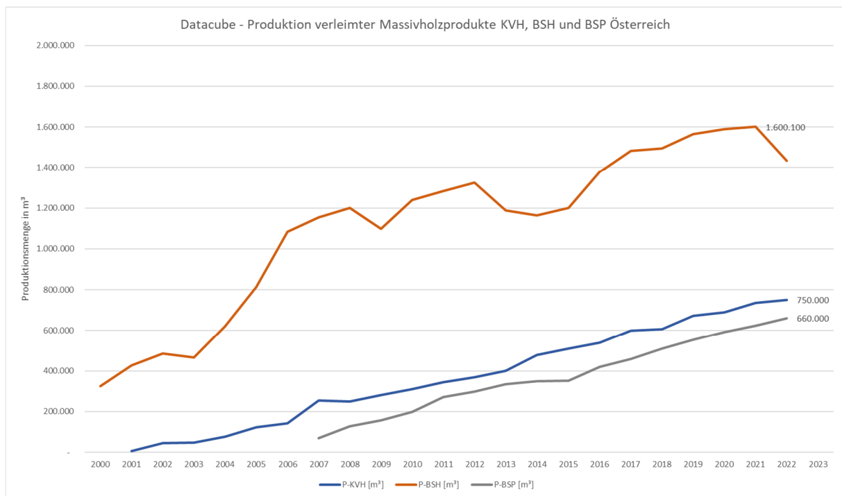
Abbildung 1 Entwicklung der Produktionsmenge (P) verleimter Massivholzprodukte, wie keilgezinktes Konstruktionsholz (KVH®), Brettschichtholz (BSH) und Brettspertholz (BSP) von 2000 bis 2022 (Quelle: Holzkurier Datacube)
