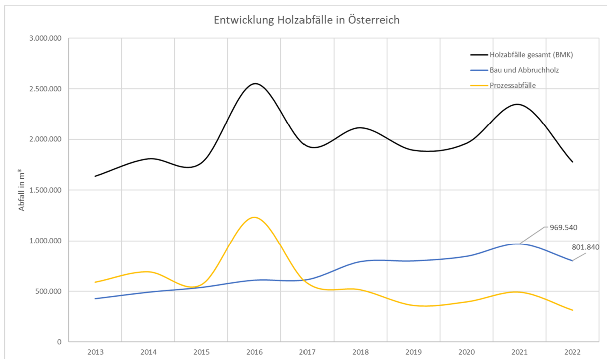
Abbildung 17 Entwicklung der Holzabfälle gesamt (schwarze Linie) der Prozessabfälle (gelbe Linie) sowie von Bau- und Abbruchholz (blaue Linie) in m 3
