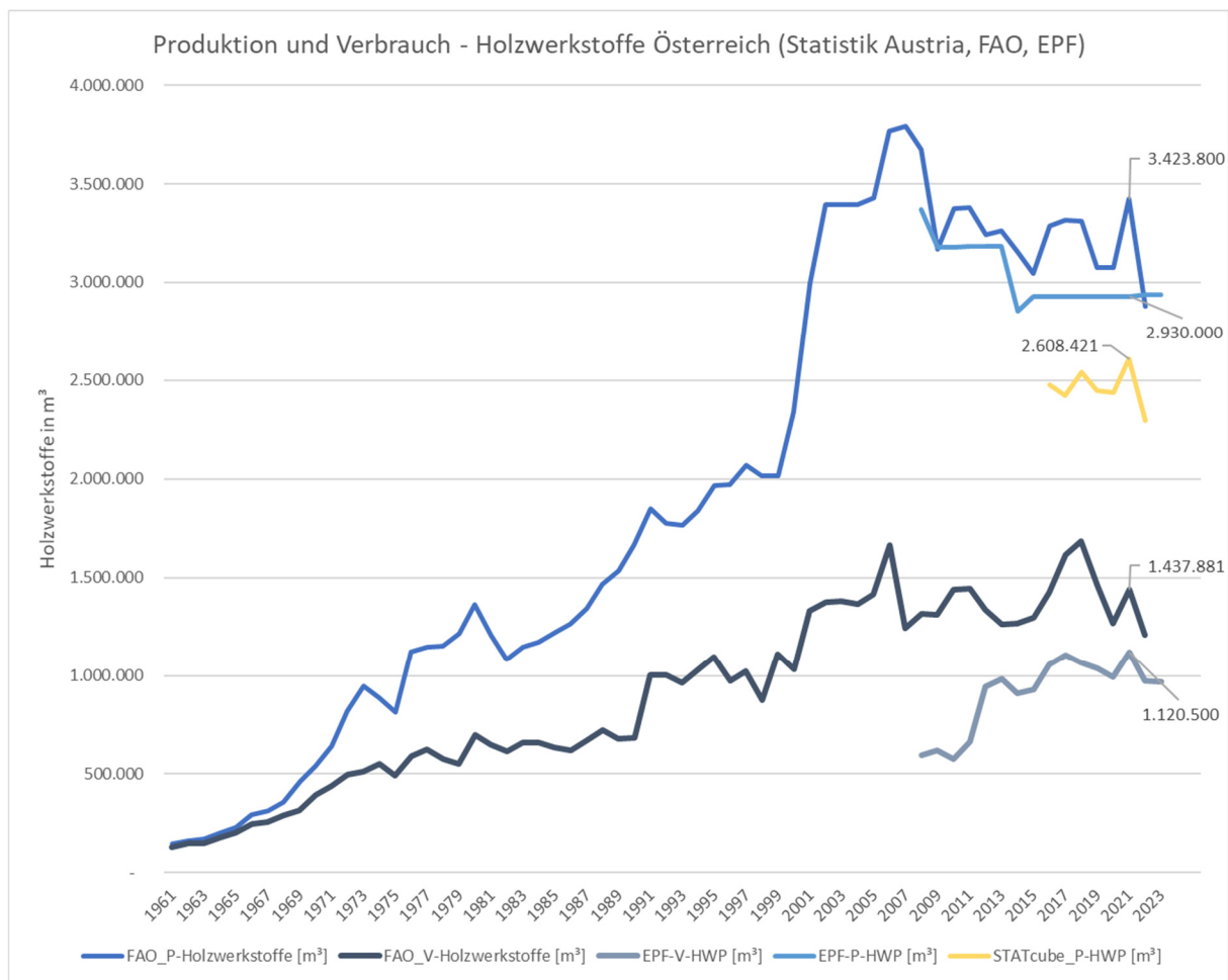
Abbildung 8 Entwicklung von Produktion (P) und Verbrauch (V) von Holzwerkstoffen entsprechend unterschiedlicher Informationsquellen (Quellen: FAO, Statistik Austria, EPF)
