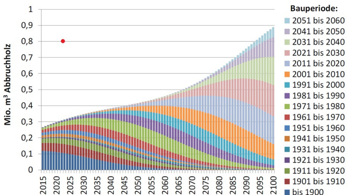
Abbildung 16 Prognostizierte Menge an Bau- und Abbruchholz in Zusammenhang mit Einwohnerentwicklung, Wohnflächennutzung und Holzbauanteil – 2015 bis 2100 [8]
